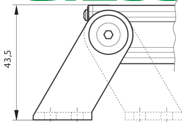
Рис.6 Габарит привода
